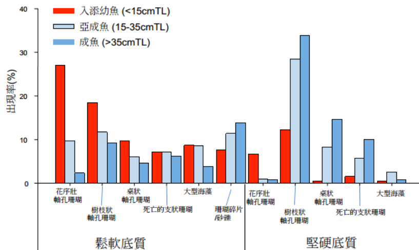
圖 3. 珊瑚礁經濟性魚類花點刺鰷( Plectropomus maculatus )在不同成長時期(體長)對於棲地喜好的選擇(modified from Wen et al. 2013a)。圖例說明：亞成魚，一年到性成熟前的個體；成魚，性成熟的個體
